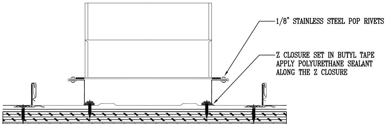
A-A SECTION
